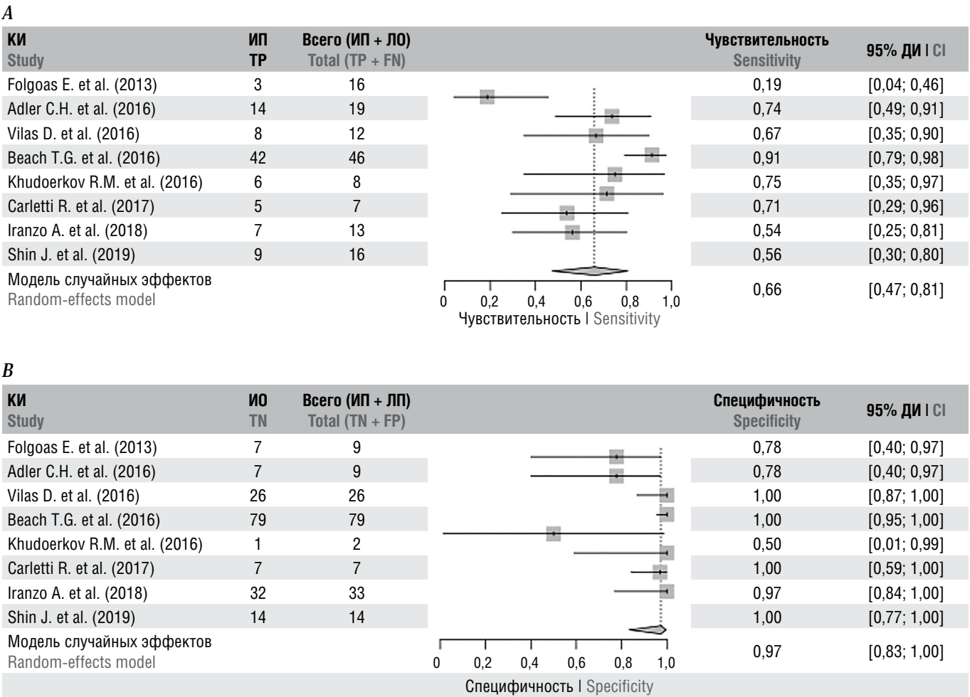
Рис. 3. Объединённая чувствительность (А) и специфичность (В) по сравнительным КИ для методов детекции \alpha -syn в СЖ пациентов с БП и в группе контроля, в которых использовались АТ к рS129- \alpha -syn. Fig. 3. Pooled sensitivity (A) and specificity (B) across the comparative studies for methods of detecting \alpha -syn in SGs of PD patients and controls using anti-pS129- \alpha -syn Abs.
