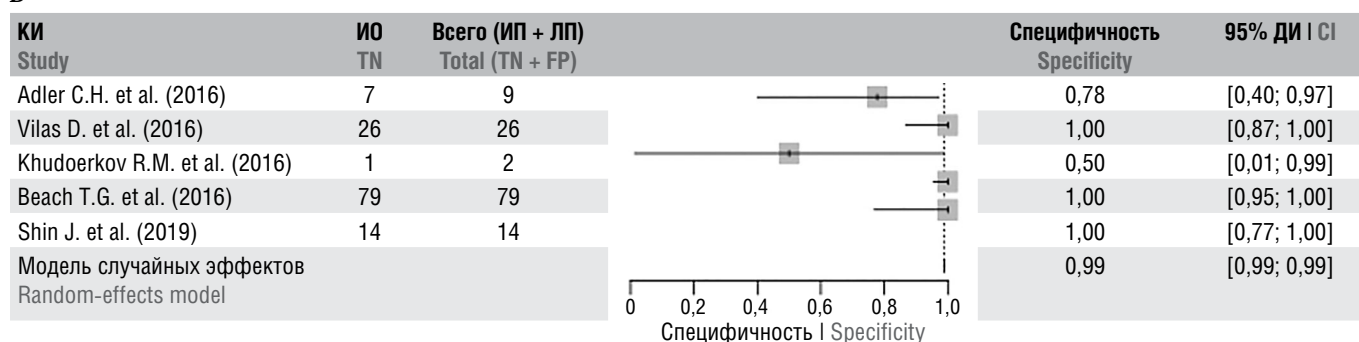
Рис. 4. Объединённая чувствительность (А) и специфичность (В) по сравнительным КИ для методов детекции \alpha -суп в СЖ пациентов с БП и в группе контроля, в которых использовались АТ к рS129- \alpha -суп и крупные СЖ в качестве материала для исследования.
